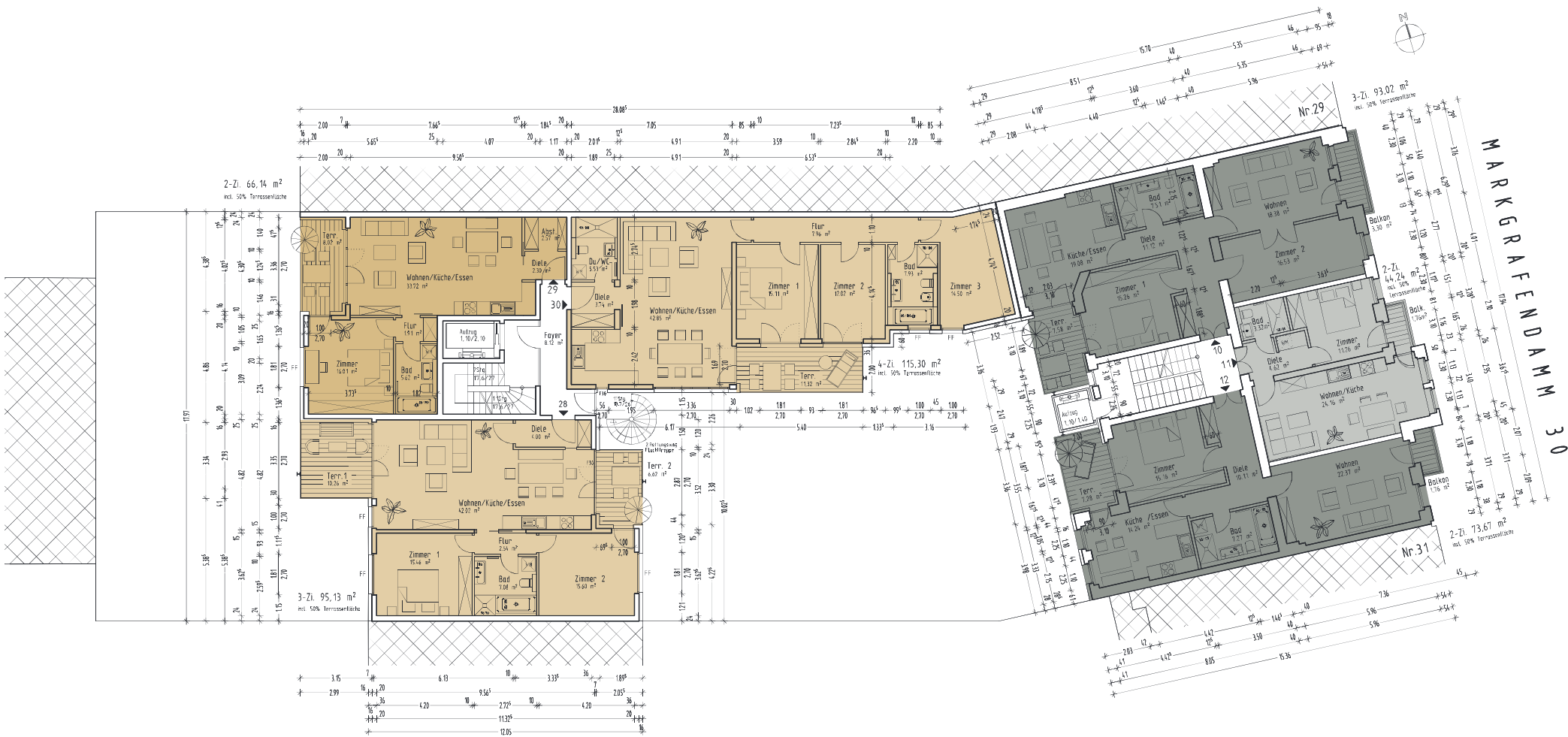
3.OBERGESCHOSS NEUBAU/ALTBAU
